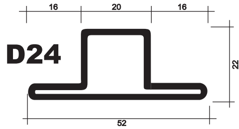
CH 16 - 4,971 Kgs/Barra CH 18 - 4,037 Kgs/Barra
