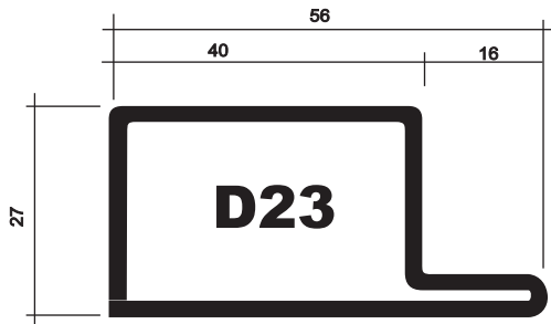
CH 16 - 5,609 Kgs/Barra CH 18 - 4,547 Kgs/Barra
