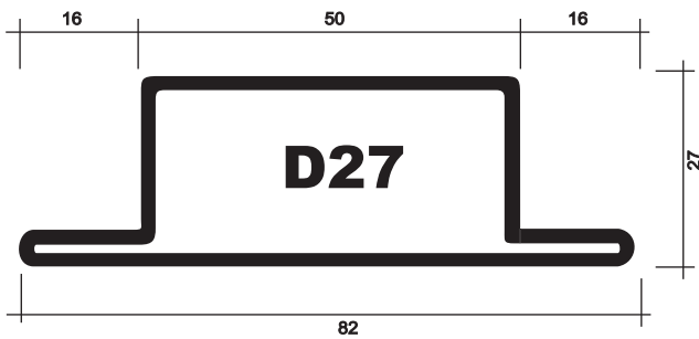
CH 16 - 7,491 Kgs/Barra CH 18 - 6,053 Kgs/Barra
