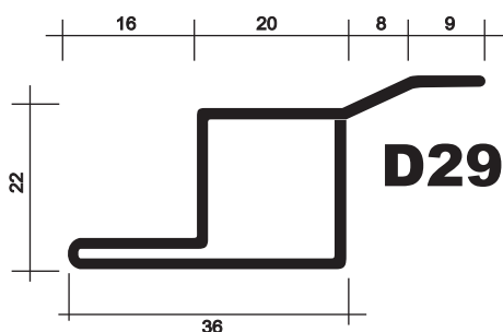
CH 16 - 4,410 Kgs/Barra CH 18 - 3,588 Kgs/Barra
